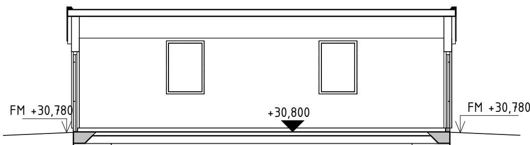
PRINCIPSEKTION A-A
