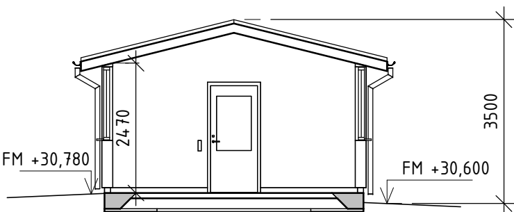
PRINCIPSEKTION B-B
